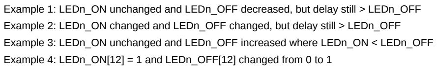
Fig 11. Update examples when LEDn_ON > LEDn_OFF
